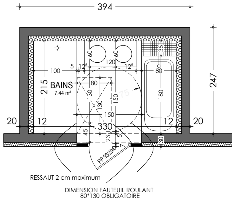
DIMENSION 330*215
