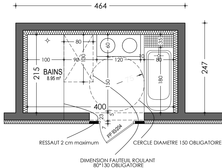
DIMENSION 400*215
